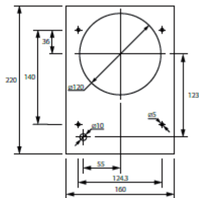
取付枠用型紙
