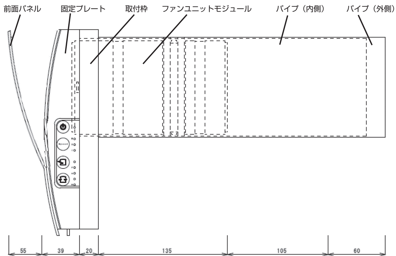
右面図
