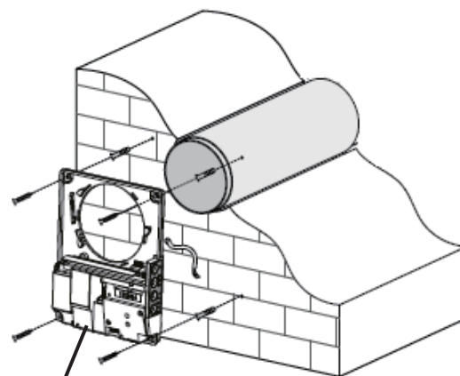
固定プレート
