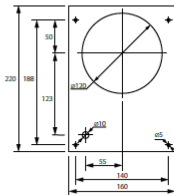
固定プレート用型紙
