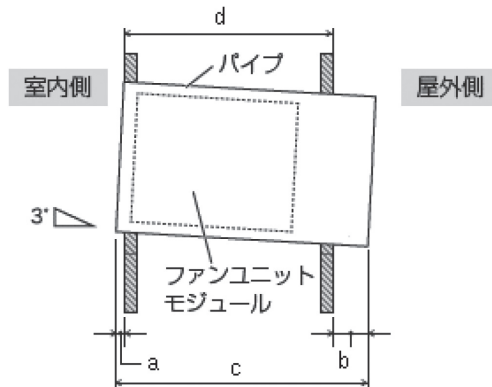
付属のパイプ・フード使用時
