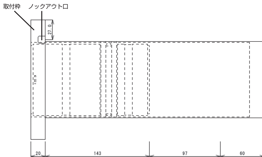
下面図
