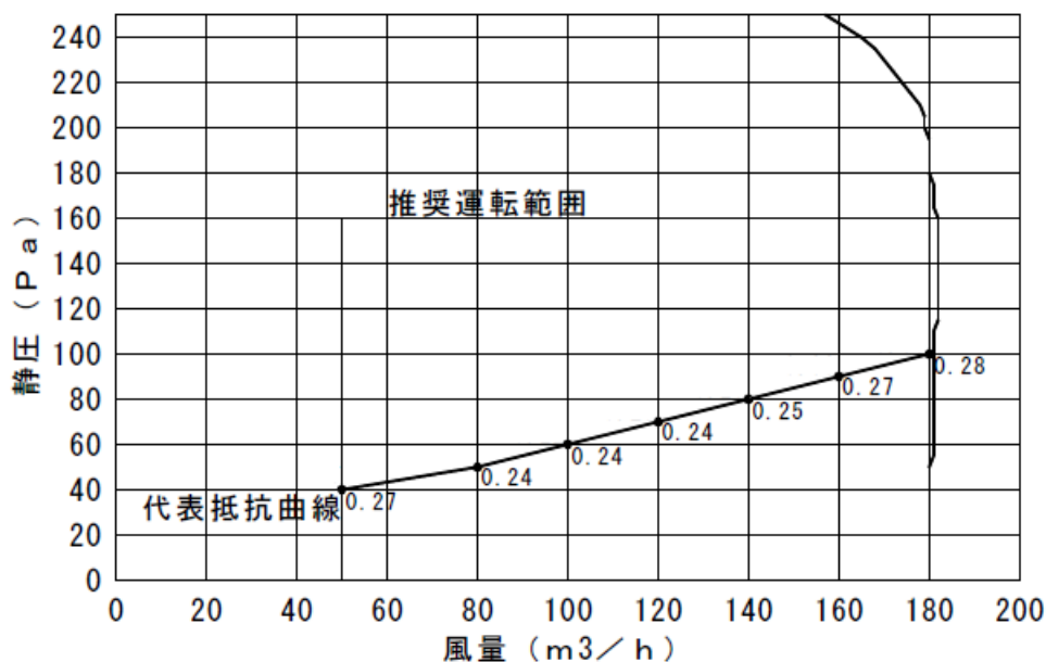
図-1 LWZ-130シリーズPQ特性図
