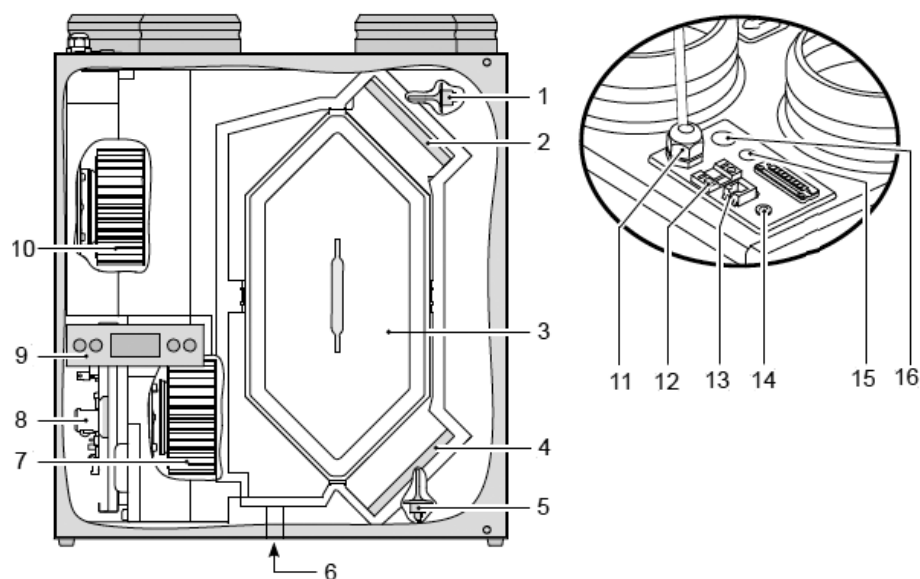
内部構成図
