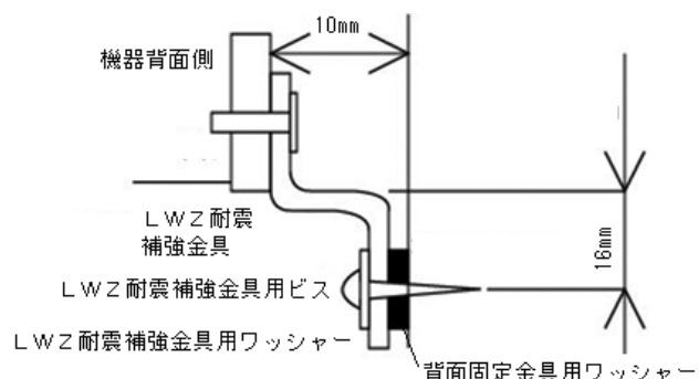
下部側面拡大図
