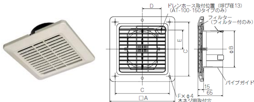
■ 変化寸法表
