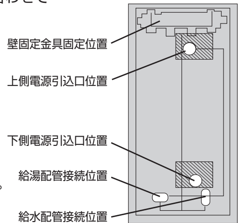
固定用型紙
