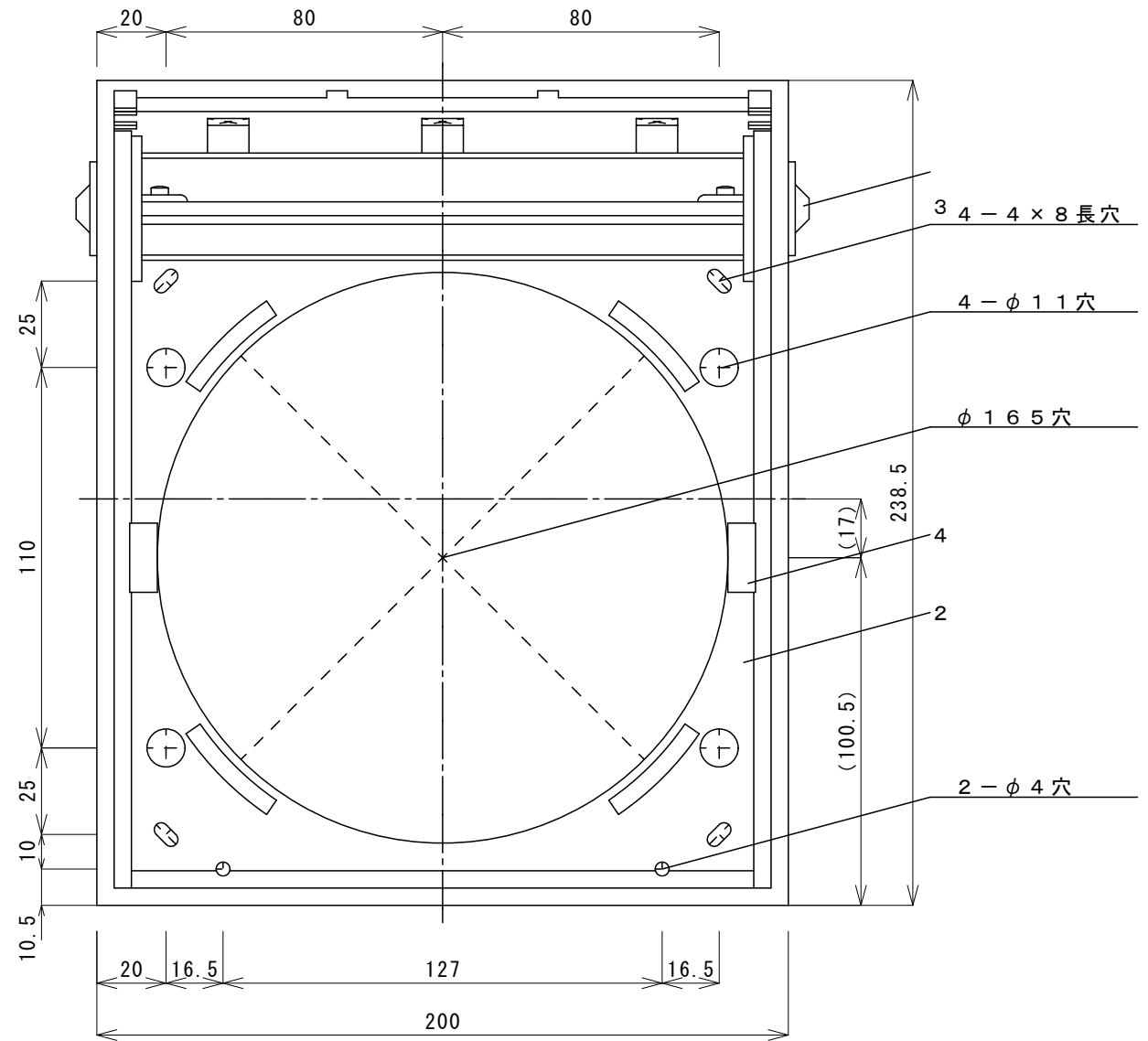
前面図
