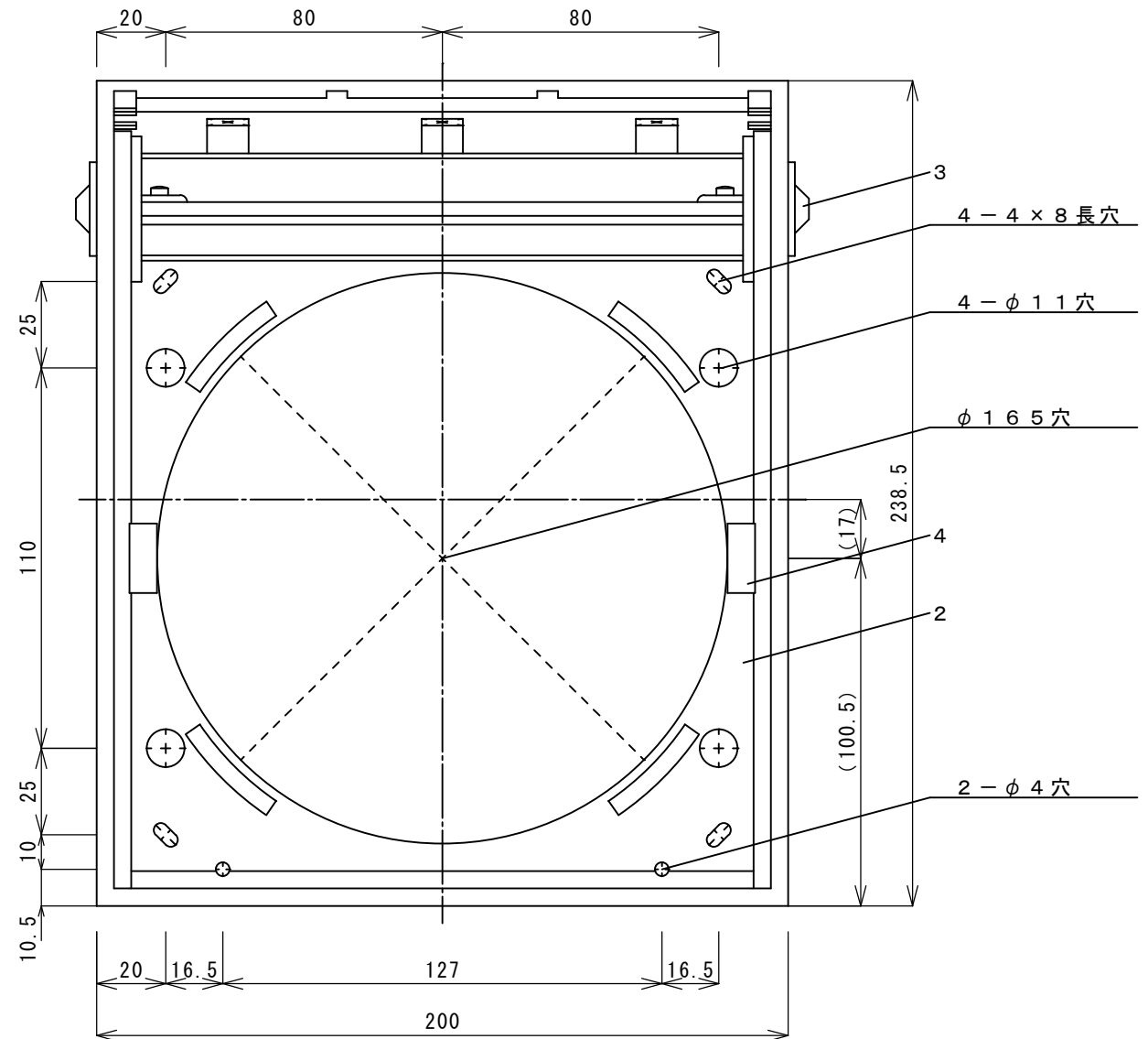
前面図
