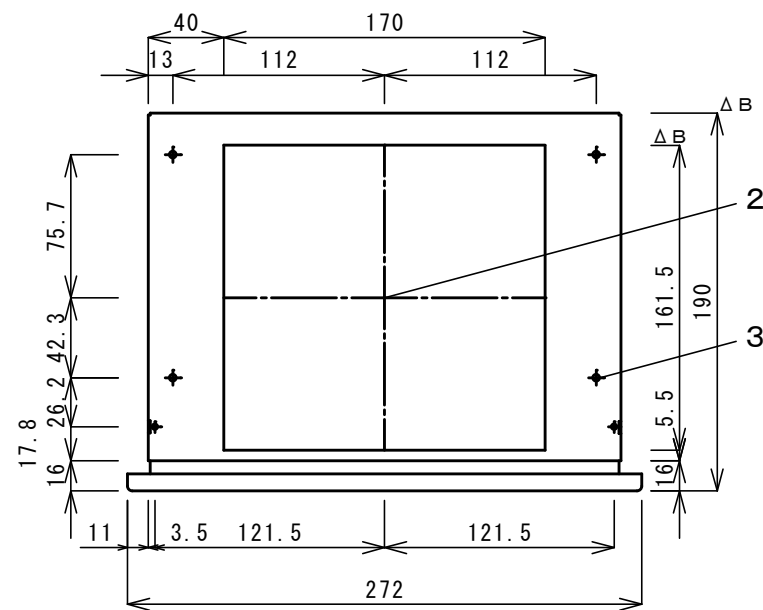
外気フード取付ベース
