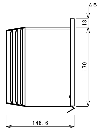
外気フード右面図
