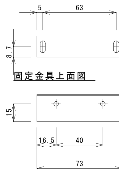
固定金具前面図
