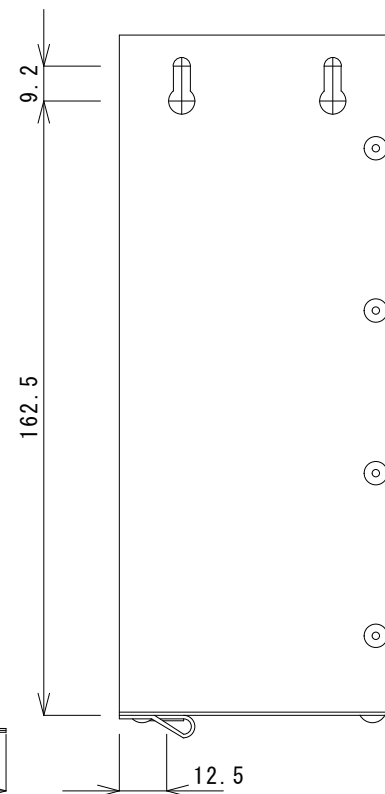
U F V - 6 0 右面図
