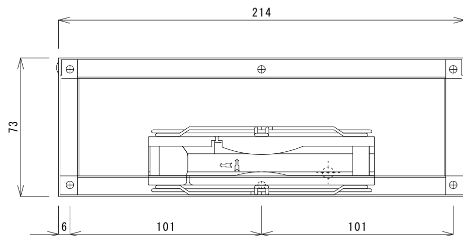
U F V - 6 0 上面図
