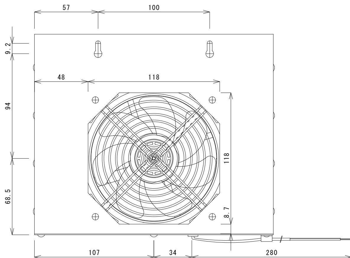
U F V - 6 0 前面図
