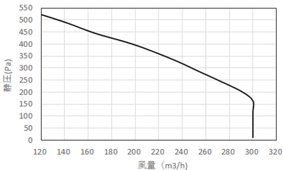
LWZ-170EPlus PQ曲線図
