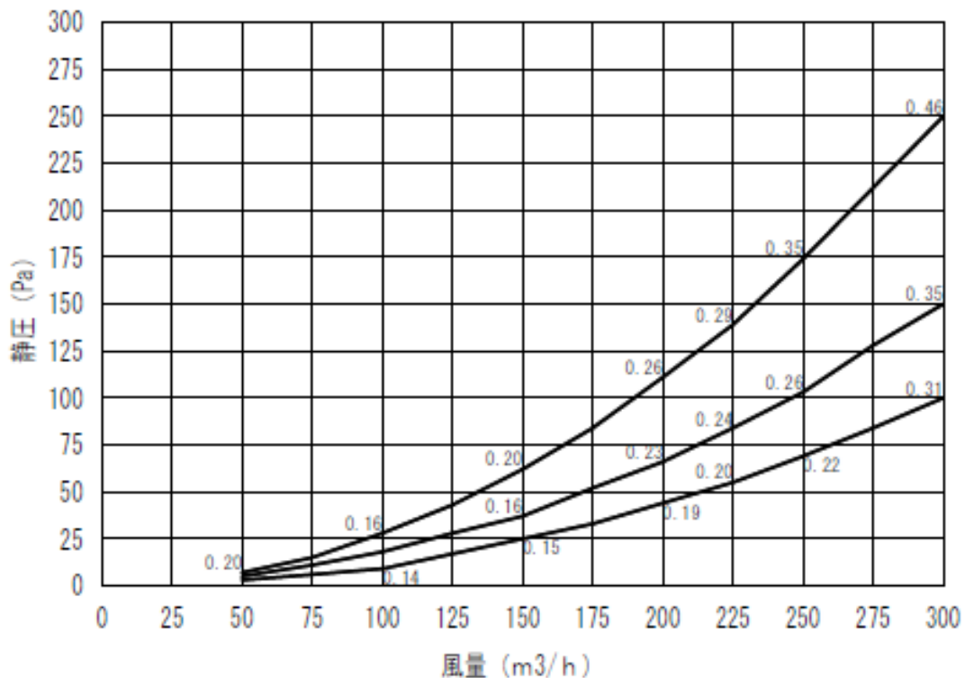
LWZ-170E Plus PQ特性図
