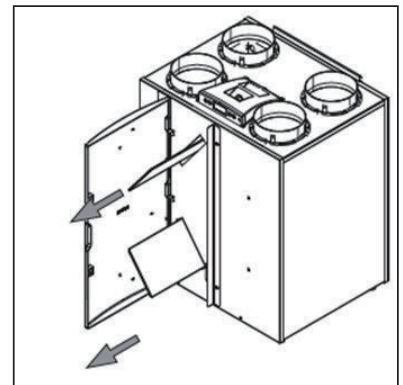
1：室内からの排気フィルター 2：室内への給気フィルター
