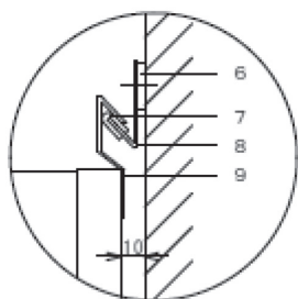
A 詳細図
