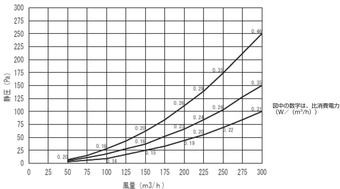
LWZ-170EPlus P-Q特性図
