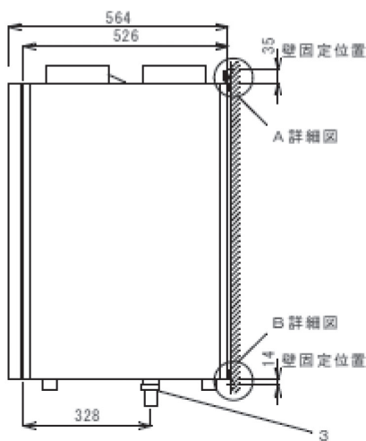
右面図
