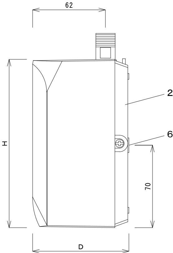
側面図
