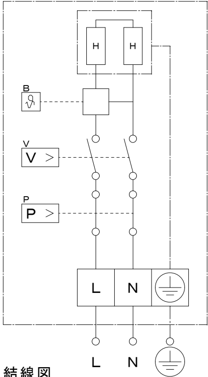
結線図
