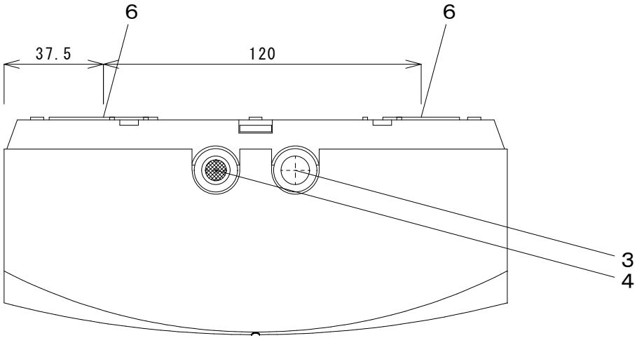
接続口面図
