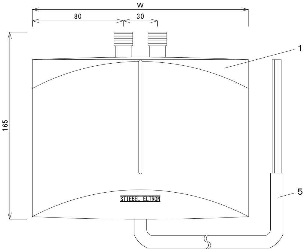
前面図
